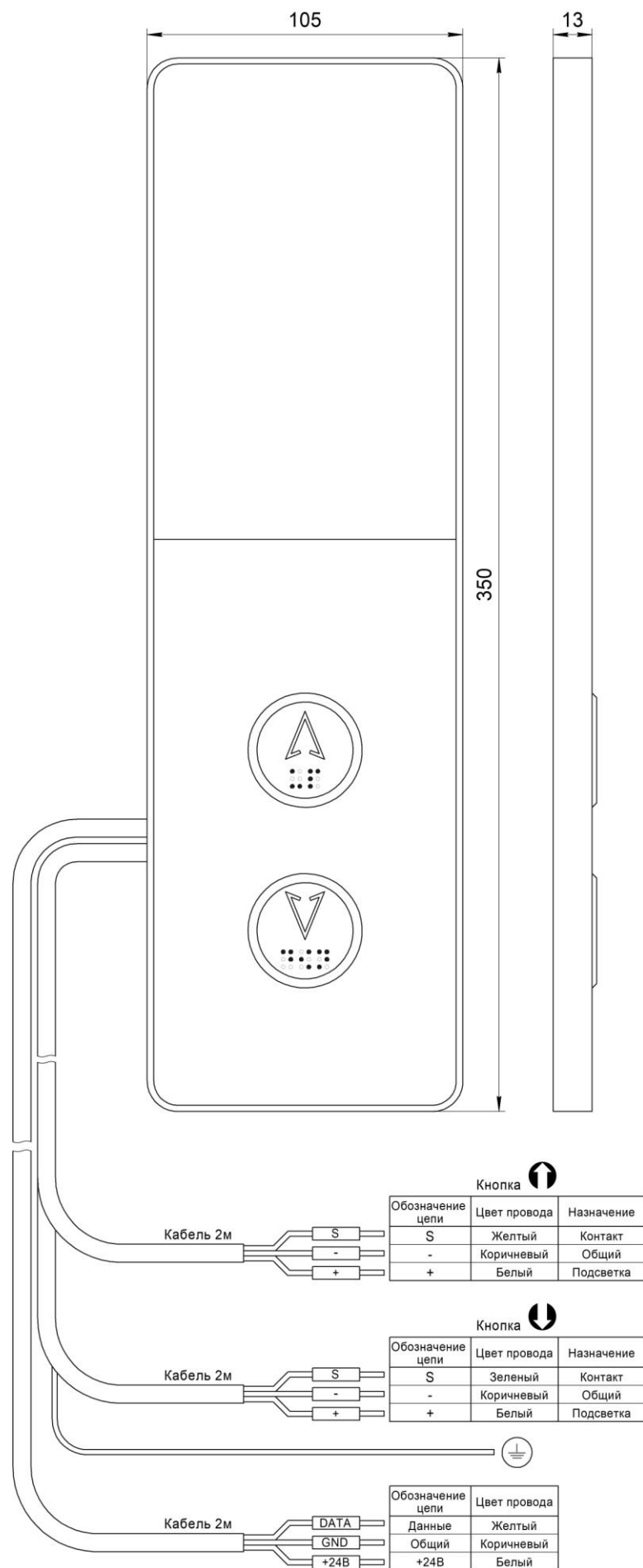
Рис.1 Внешний вид, габаритные и установочные размеры Вызывного поста МАЛАХИТ НШЕК.468381.026
